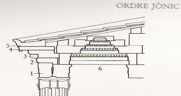
Columna i entaulament: secció (esquerra) i alçat (a dalt)
