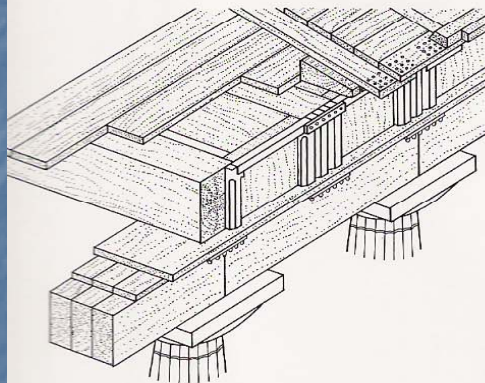
Reconstitució de l'entaulament original de fusta, del què deriva l'ordre dòric
