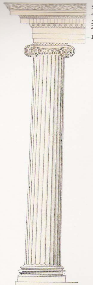
Columna i entaulament: secció (esquerra) i alçat (a dalt)
